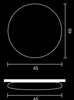
ART. 2421 Plafoniera / Ceiling lamp Plafonnier / Deckenleuchte
